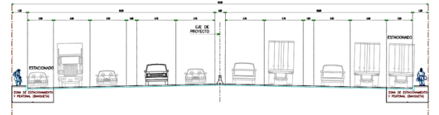
SECCION TIPICA: DERECHO DE VIA 40.00m
