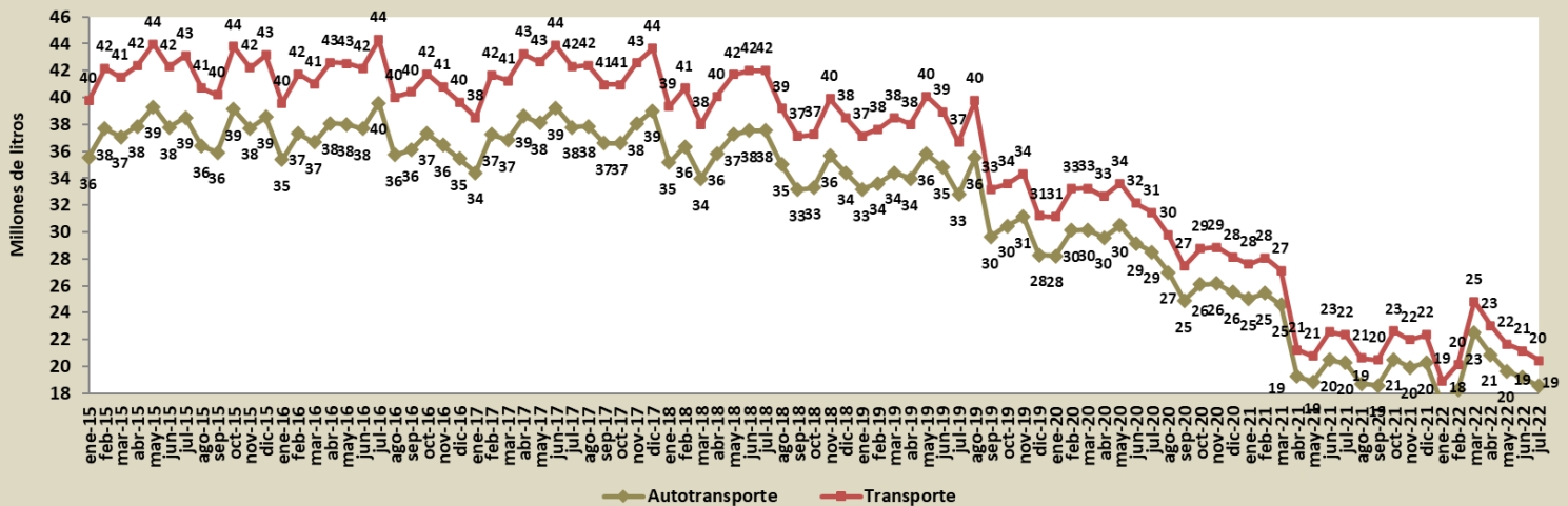
Consumo de Diesel (millones de litros diarios) 2015-2022
