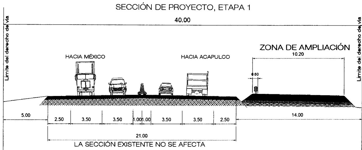
Figura no. 3.- Primera etapa de ampliación del libramiento de Cuernavaca, la circulación de vehículos no se afecta.
