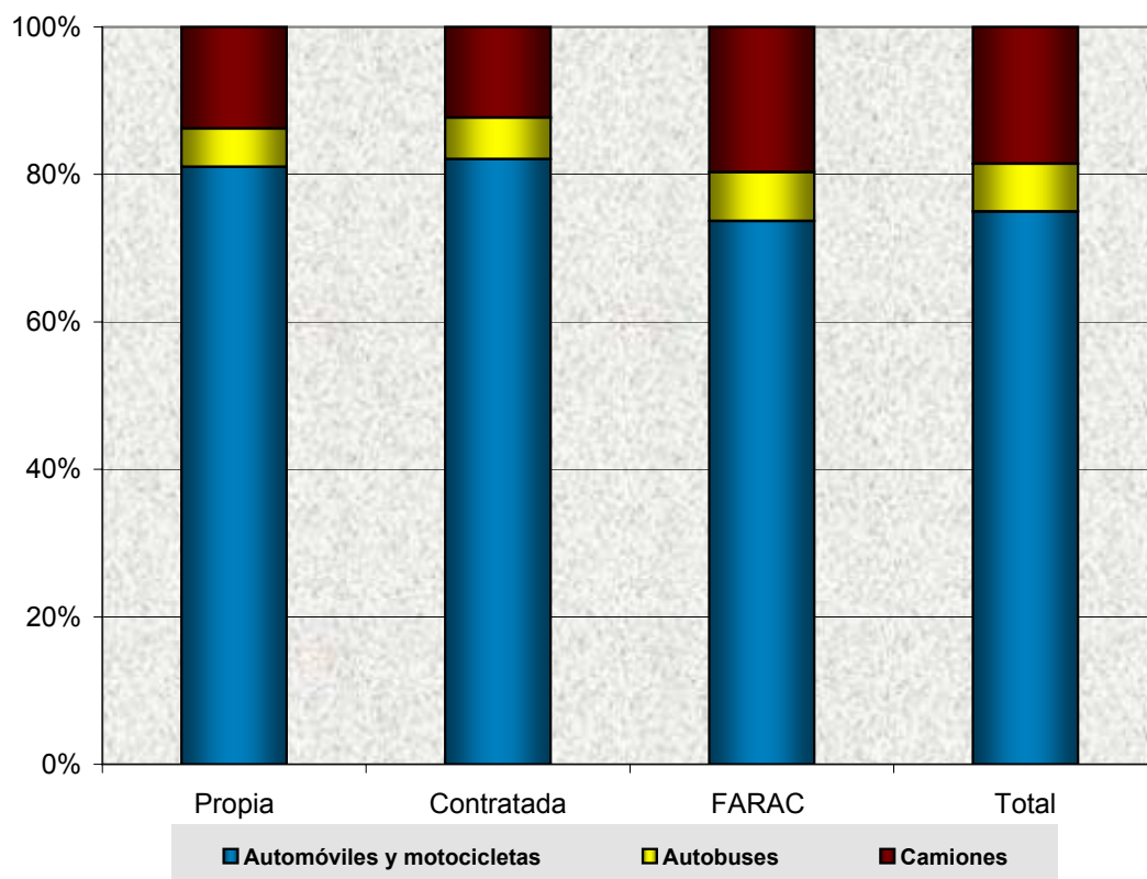
Distribución porcentual del tránsito vehicular en puentes por tipo de vehículo
