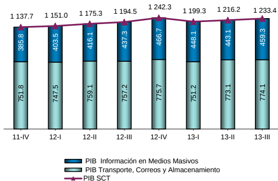
Producto Interno Bruto de Transporte, Correos y Almacenamiento e Información en Medios Masivos (Miles de millones de pesos constantes, base 100=2008) Trimestres 2011, 2012 y 2013
