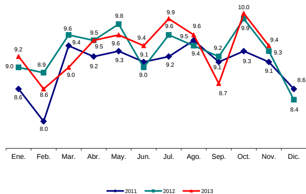
Toneladas transportadas por mes en el Sistema Ferroviario Mexicano 2011-2013 (Millones de toneladas)
