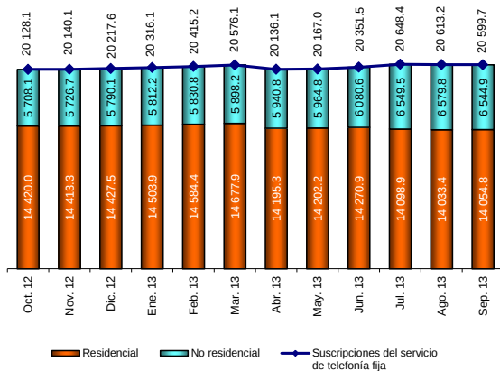
Suscripciones del servicio de telefonía fija por tipo de servicio (Miles de suscripciones)
