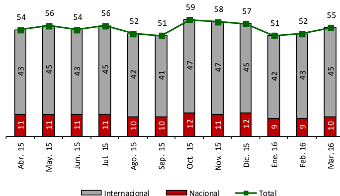
Carga transportada por las empresas aéreas (Servicio regular mensual 2015 y 2016) (Miles de toneladas)
