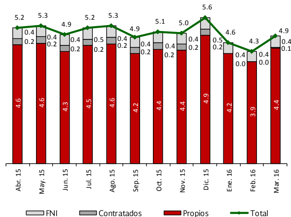
Vehículos registrados en los puentes de cuota Serie mensual de 2015 y 2016 (Millones)
