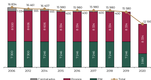
Longitud de la red de puentes de cuota a cargo de CAPUFE por tipo de red Serie anual 2006 y 2012, y de 2014 a 2020 (Metros)
