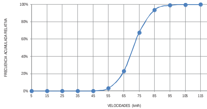
6 Carr: Querétaro - San Luis Potosí
