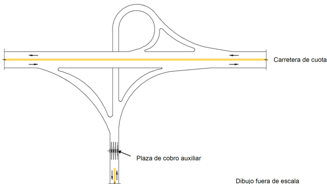
FIGURA 3.- Esquema de una plaza de cobro auxiliar (vista en planta)
