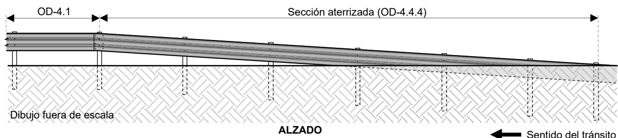
FIGURA 24.- Sección aterrizada para vigas acanaladas (OD-4.4.4)
