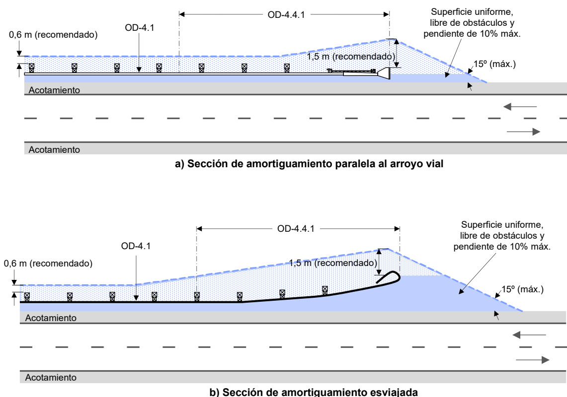
FIGURA 21.- Superficie entre el arroyo vial y la sección de amortiguamiento (OD-4.4.1)
