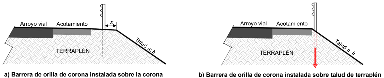
FIGURA 8. Instalación de barrera de orilla de corona (OD-4.1) en terraplén o balcón
