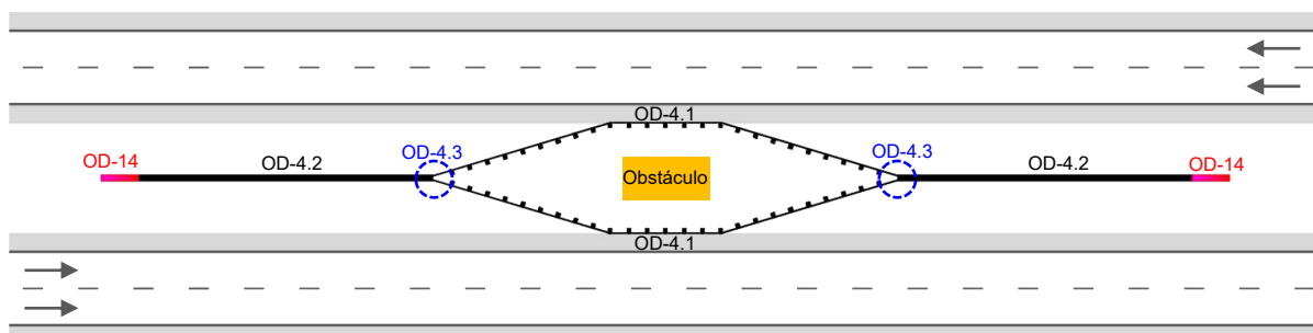
FIGURA 18.- Emplazamiento longitudinal de barreras separadoras de sentidos de circulación (OD-4.2)
