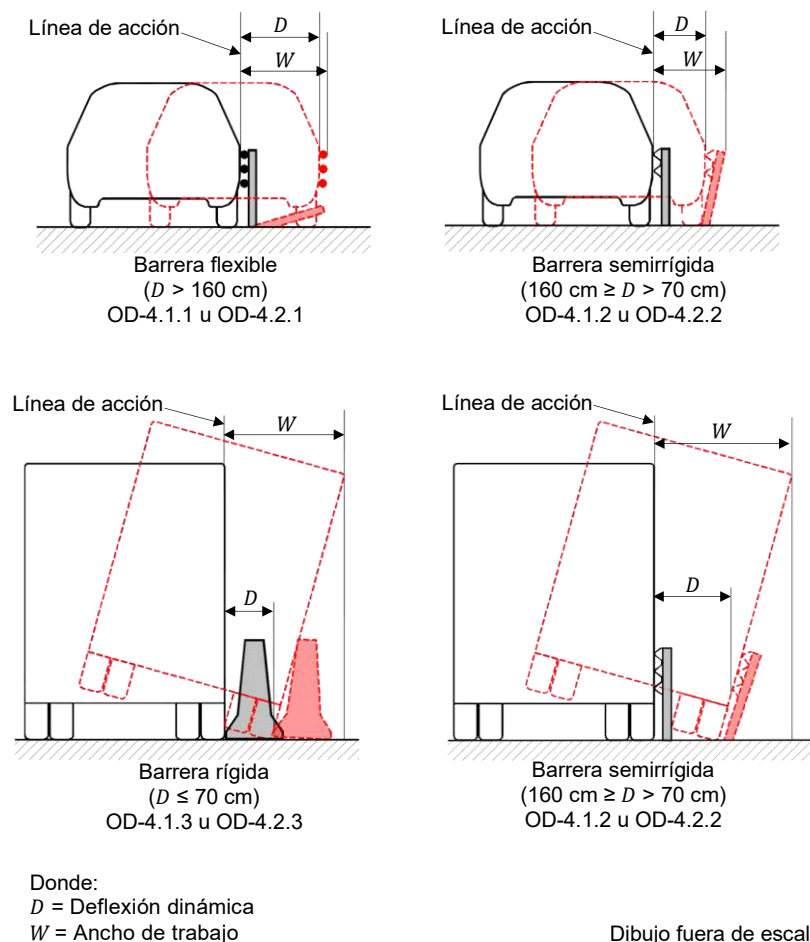
FIGURA 1.- Deflexión dinámica y ancho de trabajo de diferentes tipos de barreras de protección (OD-4)
