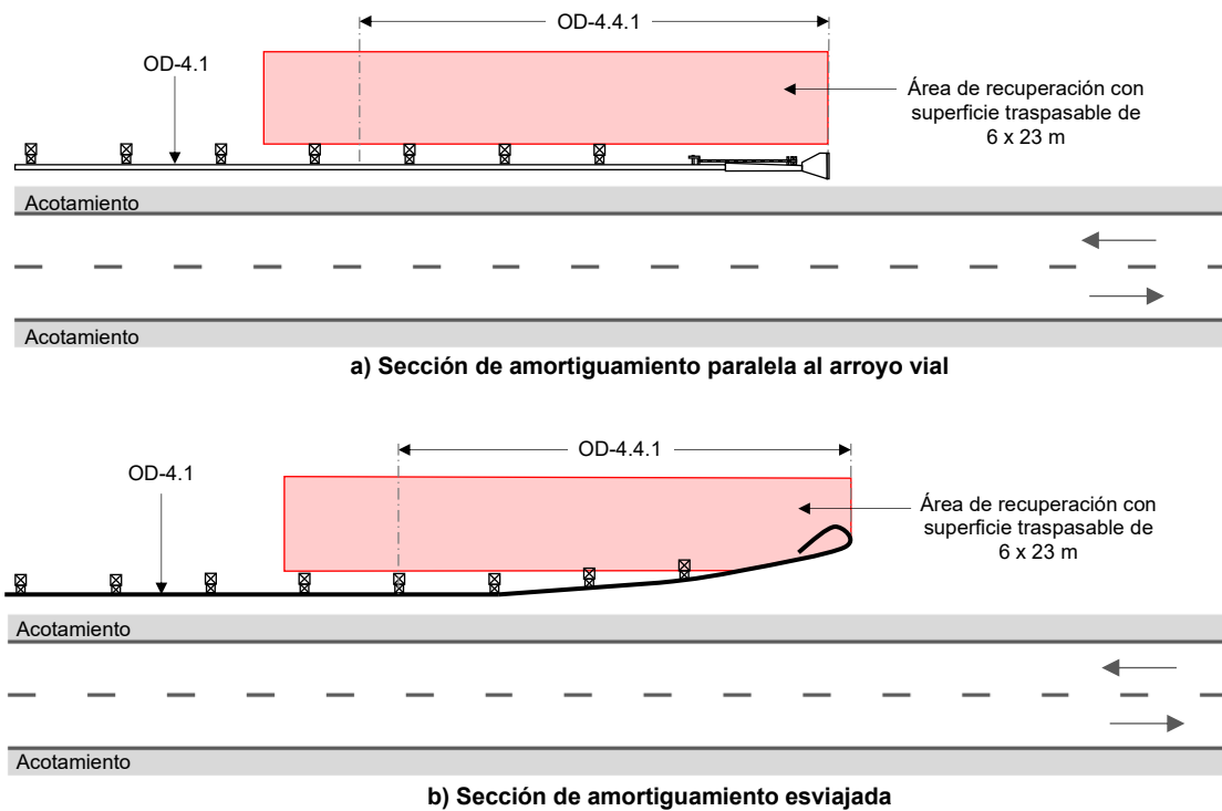
FIGURA 22.- Área de recuperación detrás y más allá de la sección secciones de amortiguamiento (OD-4.4.1)
