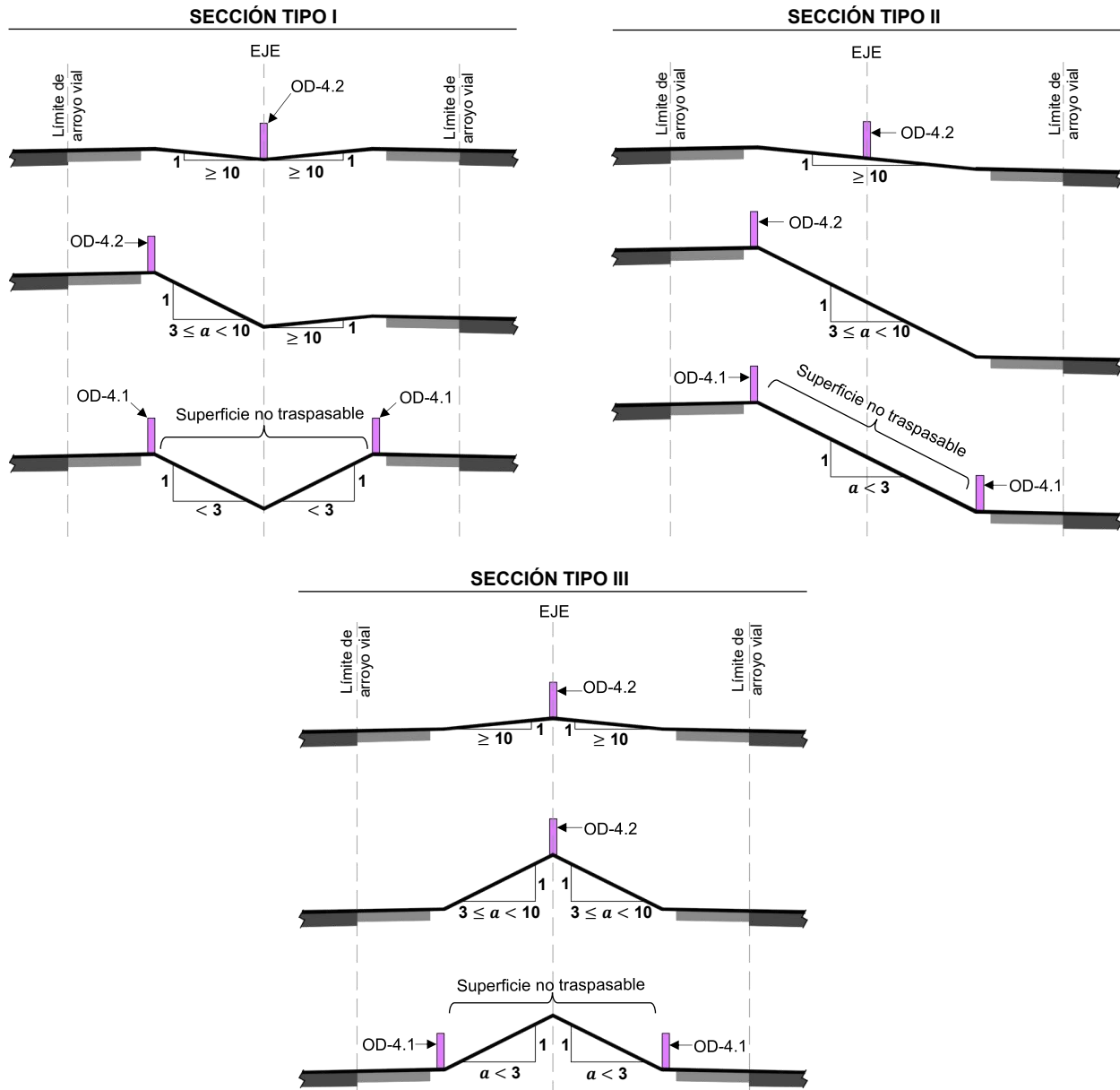
FIGURA 7. Consideraciones para diferentes tipos de secciones en la faja separadora central
