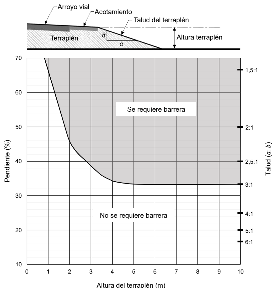
FIGURA 2.- Necesidad de barreras de orilla de corona (OD-4.1) en terraplenes y balcones
