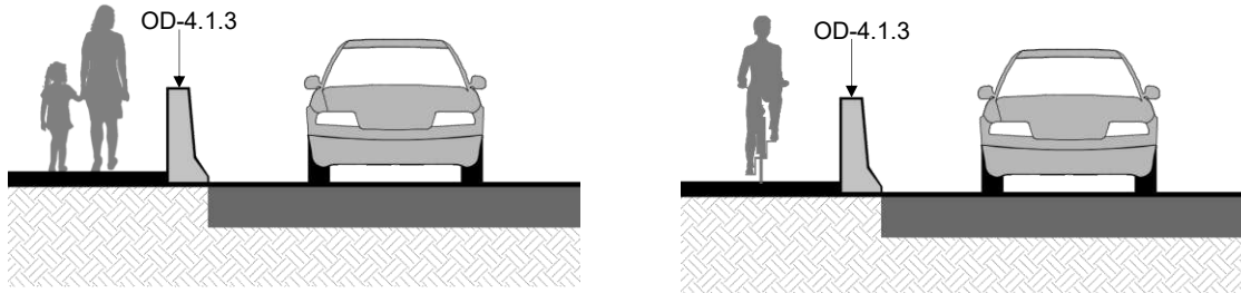
FIGURA 3.- Utilización de barreras de orilla de corona (OD-4.1) para proteger peatones y ciclistas
