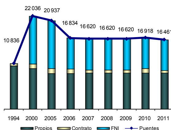
Longitud de la Red de Puentes de CAPUFE (Metros)
