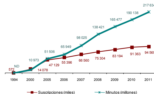
Suscripciones y minutos de telefonía móvil
